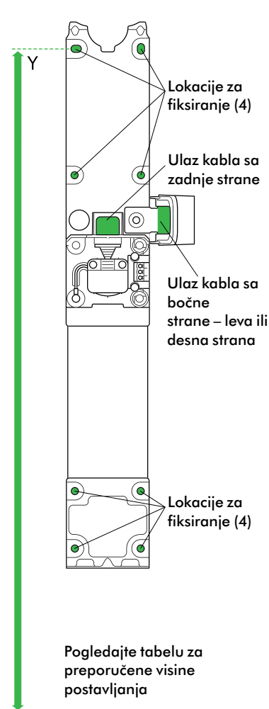
Montažna ploča
